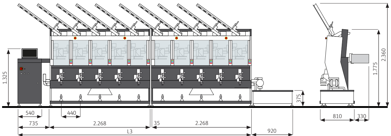
Silindir yüzeyinden soğuk yağlama sistemi PU11
